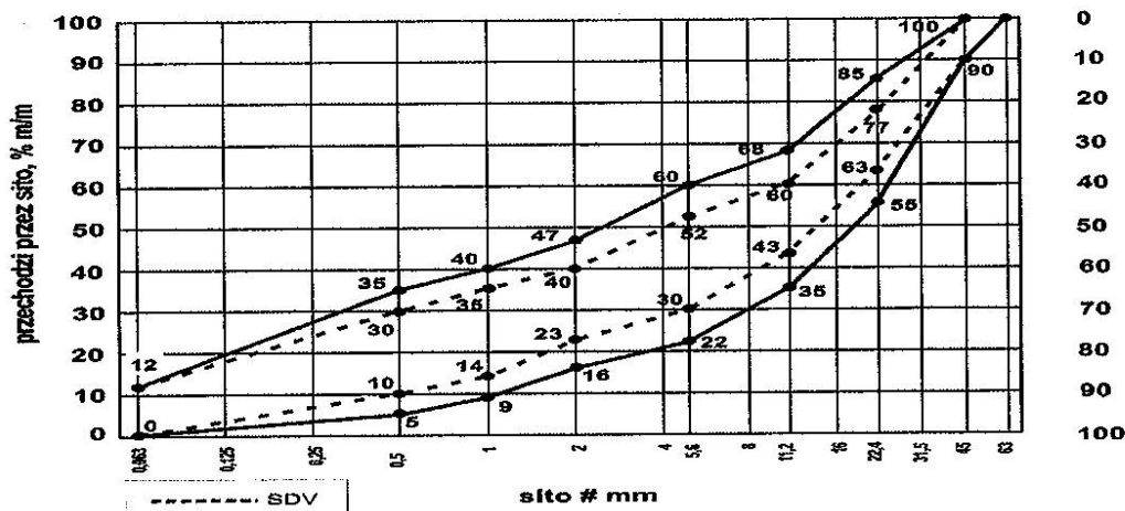
Rysunek 1. Mieszanka niezwiązana 0/45 do warstwy podbudowy pomocniczej
