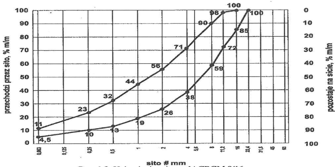
Rys. 1.3. Uziarnienie mieszanki CBGM 0/16
