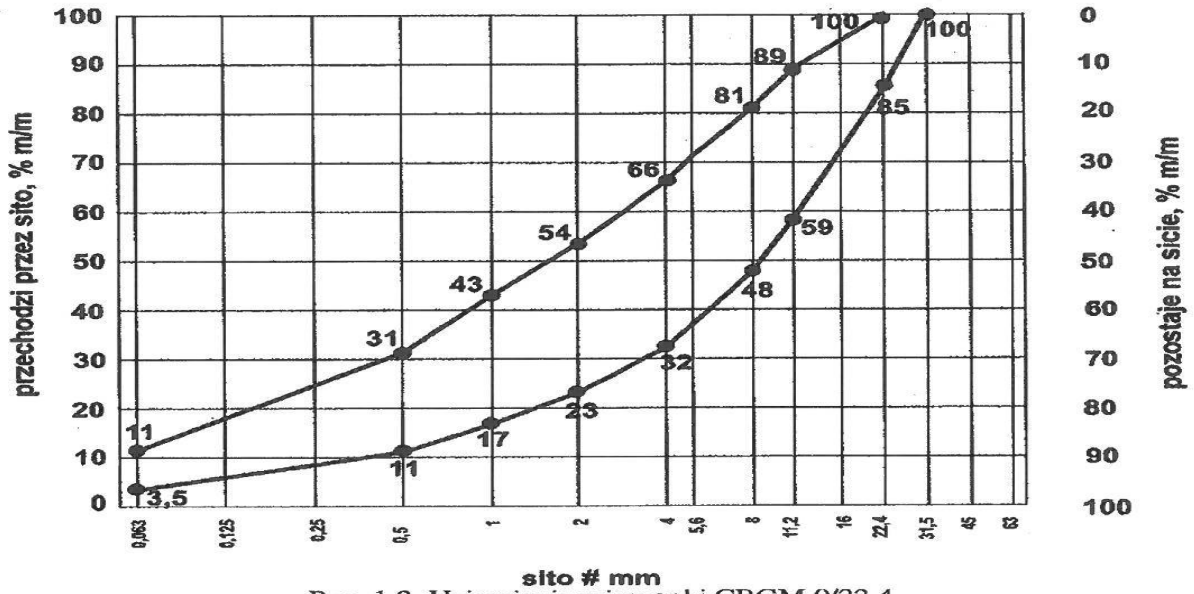
Rys. 1.2. Uziarnienie mieszanki CBGM 0/22,4
