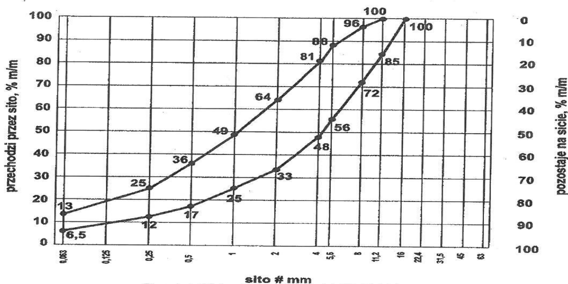
Rys. 1.4. Uziarnienie mieszanki CBGM 0/11,2
