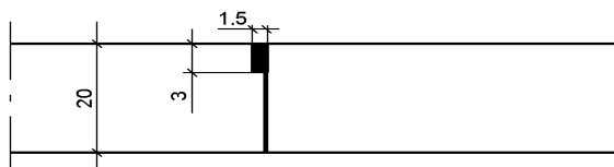
Rys. 1.1. Przykłady konstrukcji szczelin w podbudowie z betonu cementowego (wymiary w cm)
