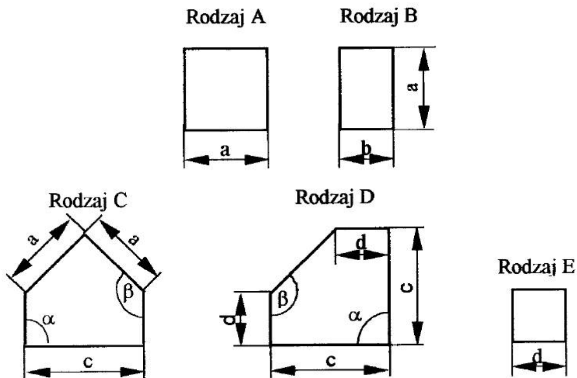
Rysunek 1. Rodzaje płyt chodnikowych betonowych
